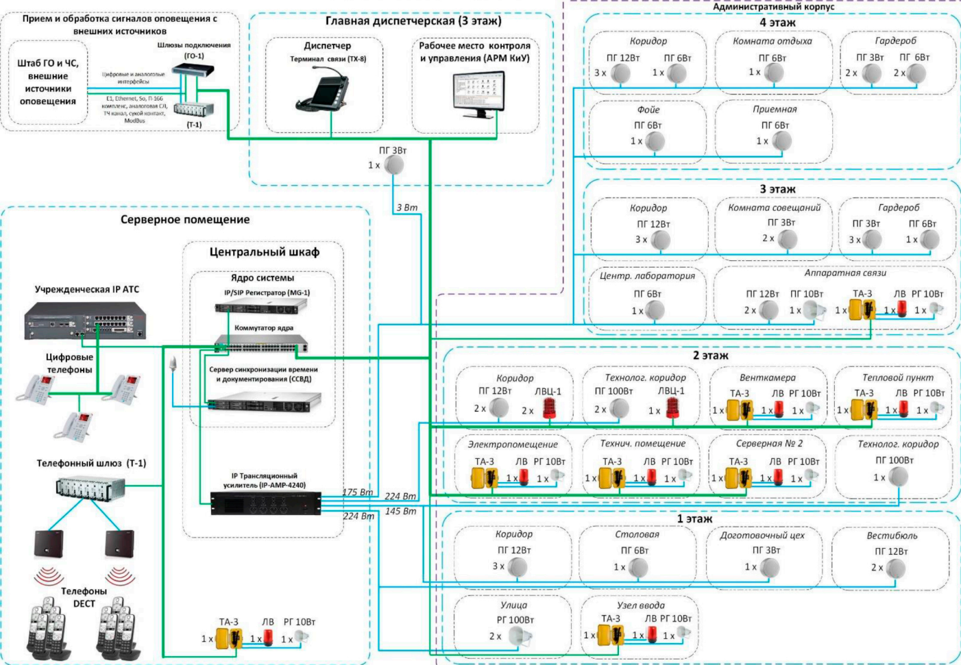
Схема системы диспетчерской громкоговорящей связи, оповещения и музыкального вещания промышленного объекта
