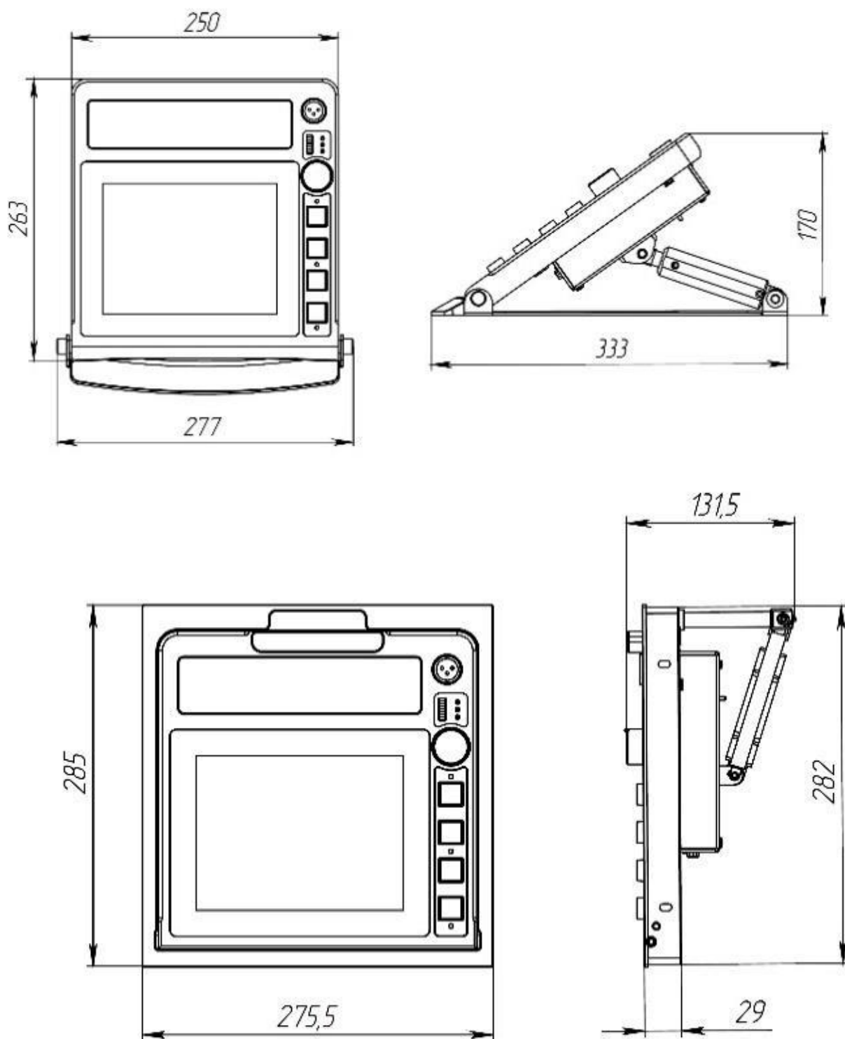
Рисунок 1. Габаритные размеры TSDT-8
